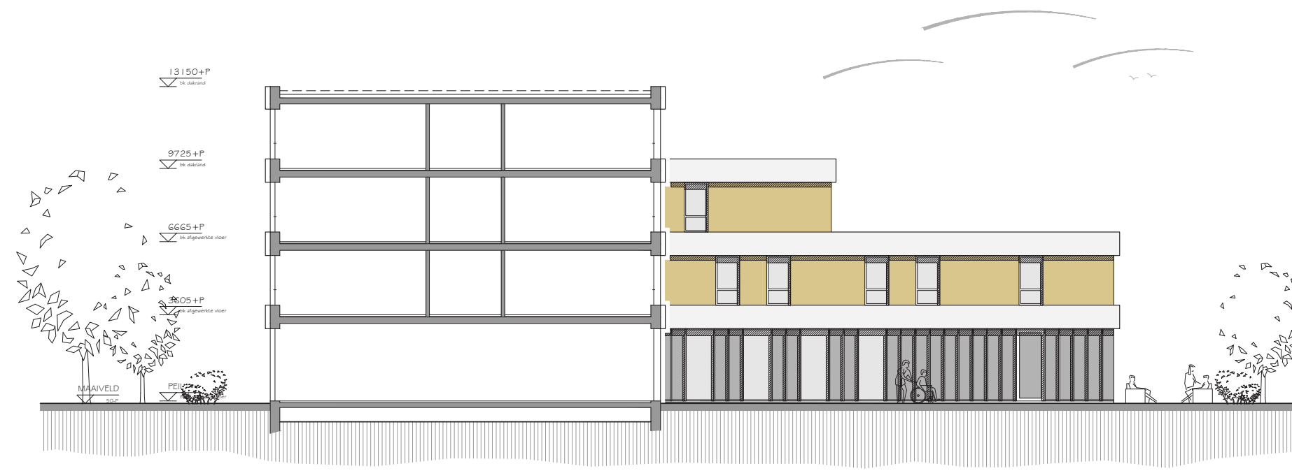
NOORDGEVEL (BINNENRUIMTE)
